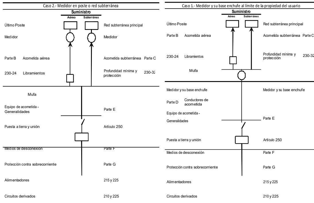
Figura 230-1.- Acometidas
